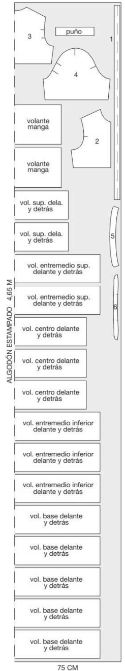
PLANO DE CORTE
