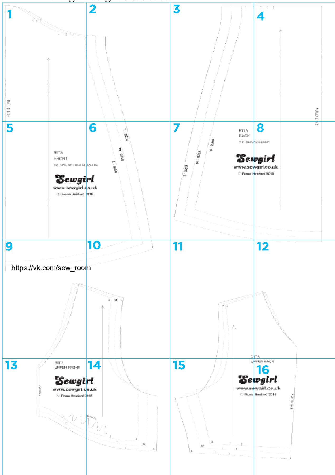
Ночная рубашка с кружевом, схема склейки
